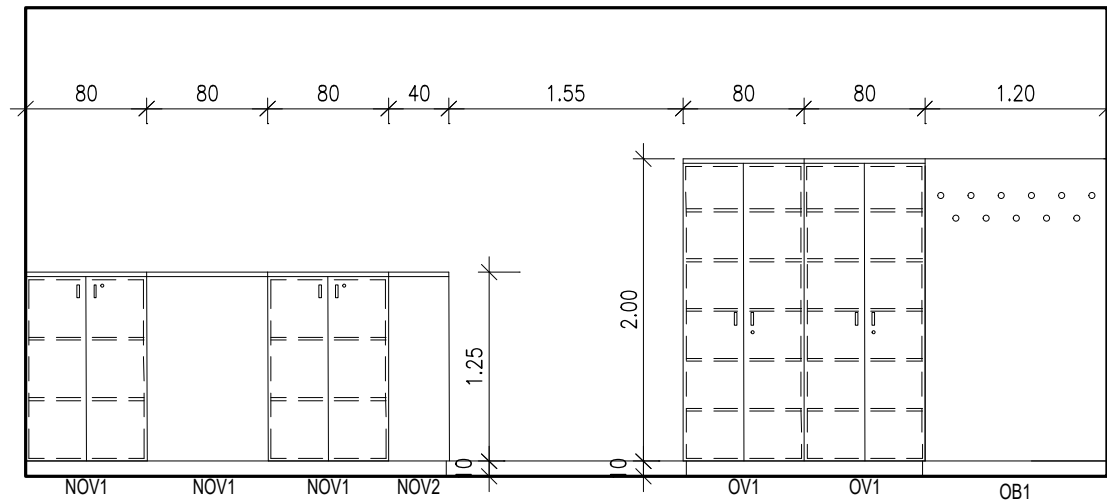
POGLED C
