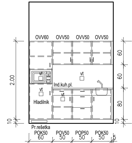
POGLED E
